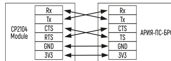
Рис.1. Схема подключения программатора CP2104 к блокам речевого оповещения серии АРИЯ-ПС-БРО.
