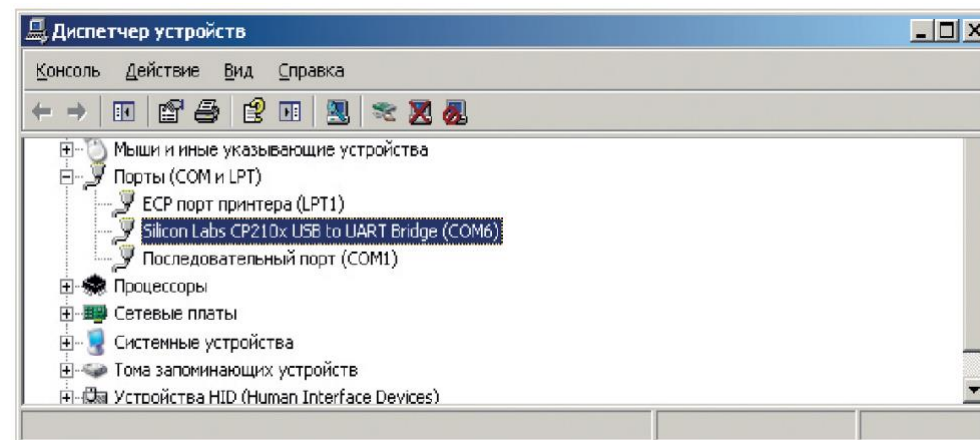
Рис.2. Диспетчер устройств.
