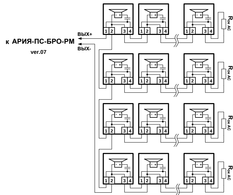
Г. Схема соединений 8, 12, 16, 20, 24, 28, 32, 36, 40, 44 и 48 речевых оповещателей серии АРИЯ-ПС.
