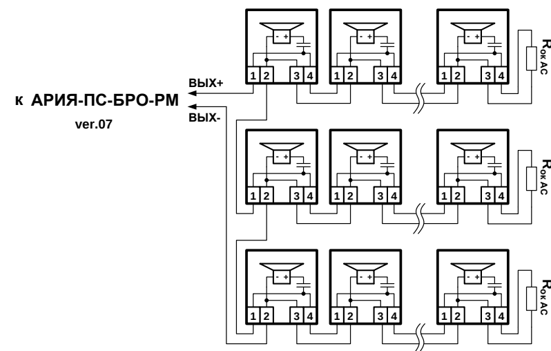
В. Схема соединений 6, 9, 12, 15, 18, 21, 24, 27, 30, 33 и 36 речевых оповещателей серии АРИЯ-ПС.
