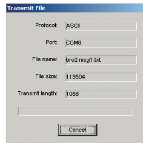
Рис. 9. Запись файла.
